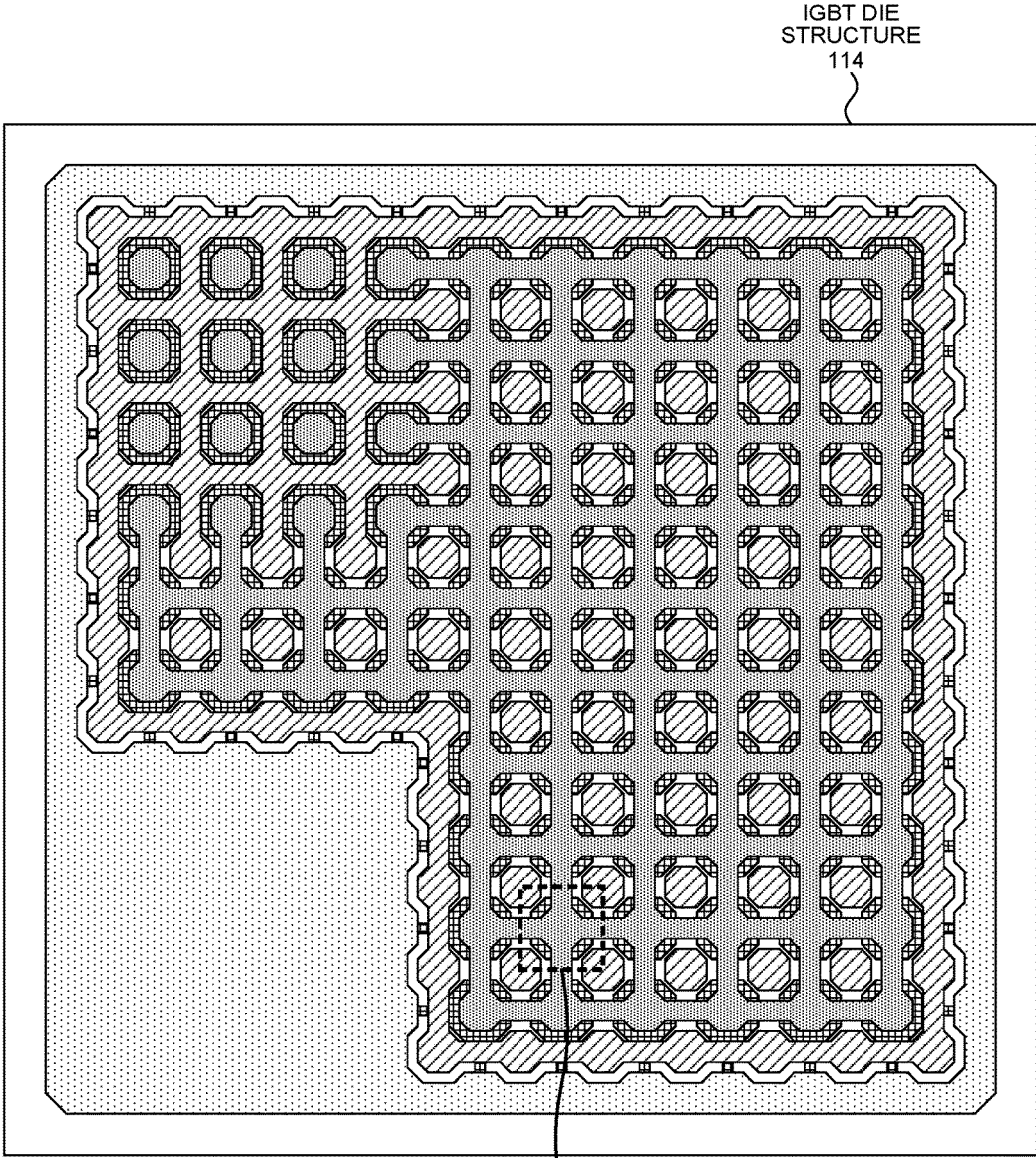
UNIT CELL 108 OF FIGS. 9A-14A
