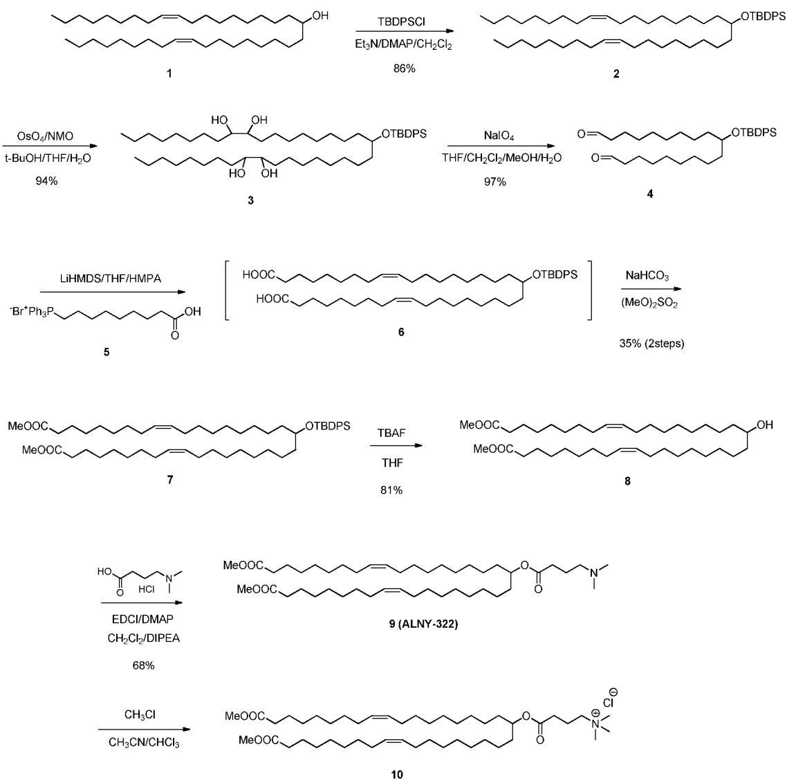
Scheme 1. ALNY-322/quaternary salts
