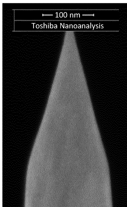
SEM image
