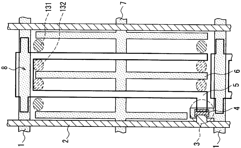
FIG. 13A (Feeding Side)
