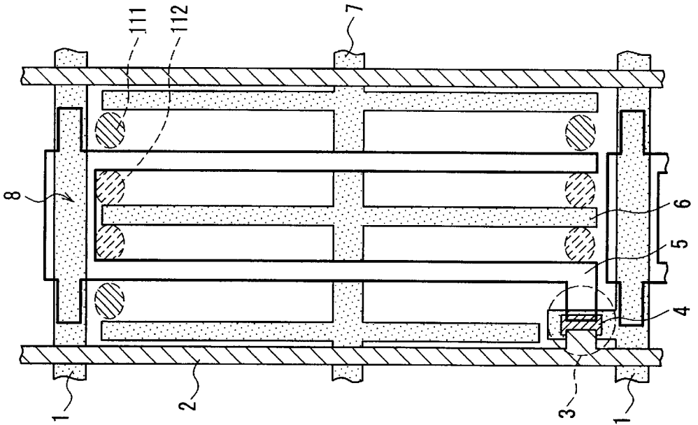
FIG. 11A (Feeding Side)
