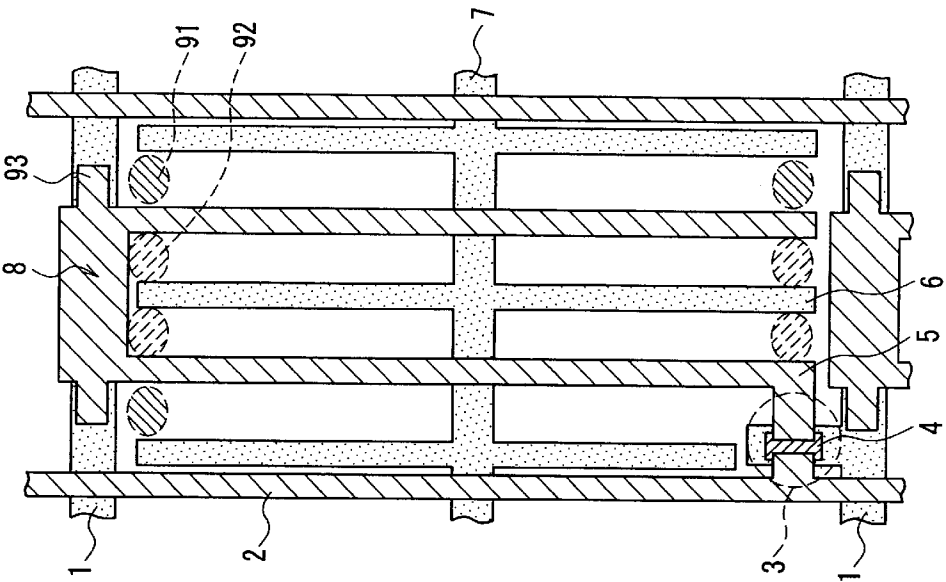
FIG. 10A (Feeding Side)
