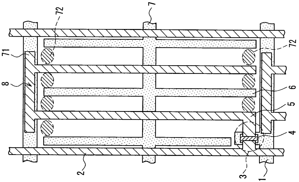
FIG. 7A (Feeding Side)
