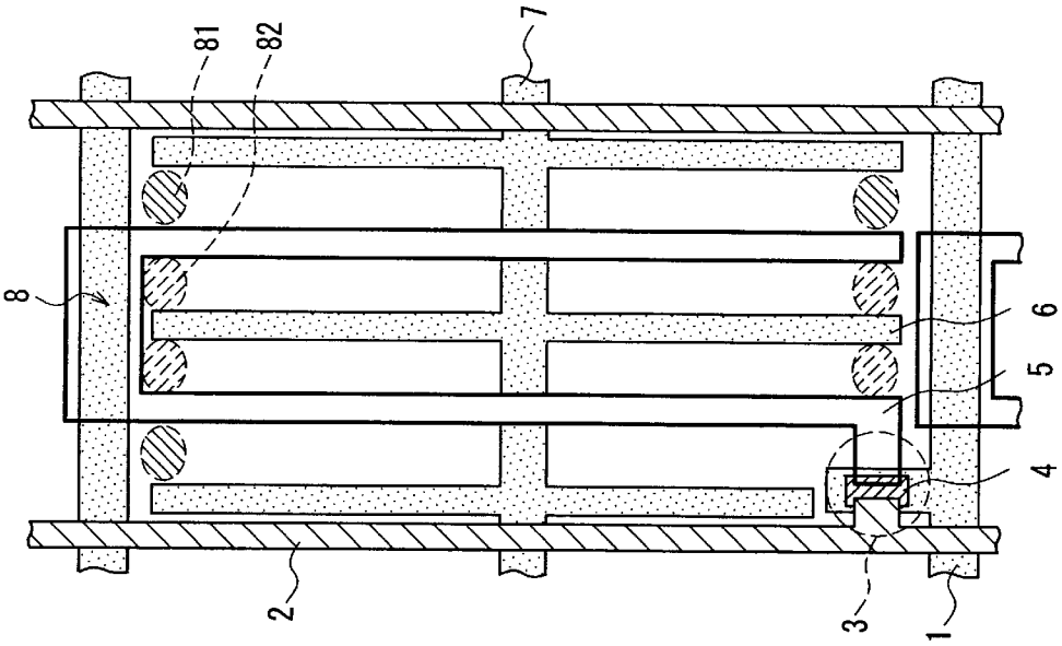
FIG. 8A (Feeding Side)
