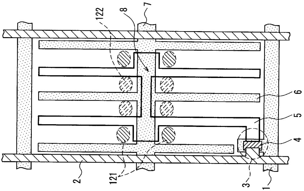
FIG. 12A (Feeding Side)
