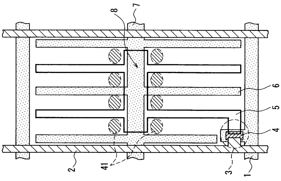
FIG. 4A (Feeding Side)
