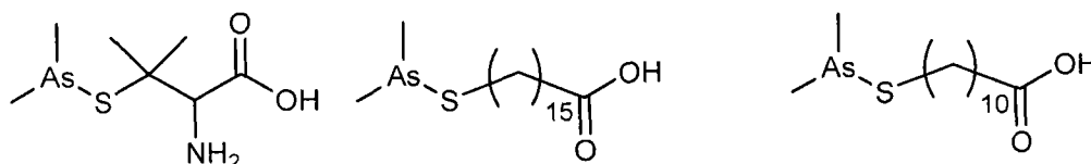
[0140] 化合物 D
