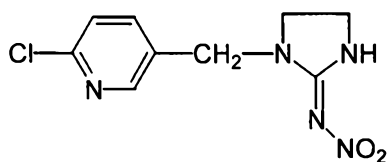
Imidacloprid
