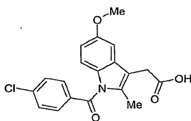
Indomethacin
