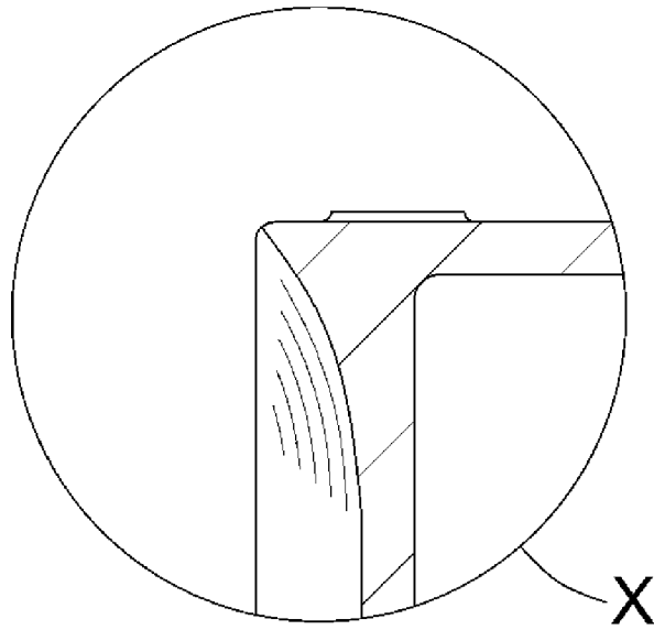
【局部放大圖】
