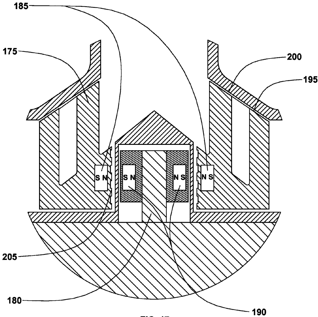
FIG. 17 (DETAIL E)
