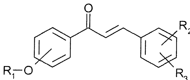
[chemische Formel 2]
