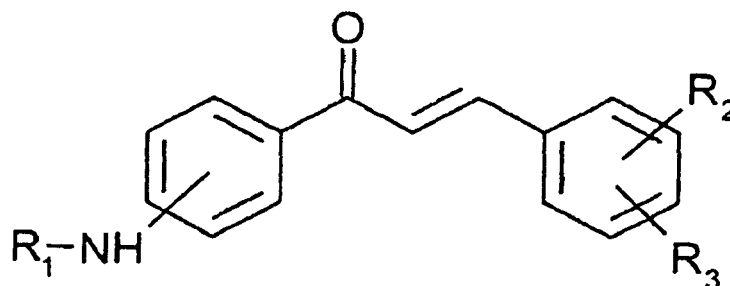
[Formule chimique 1]
