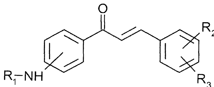
[chemische Formel 1]
