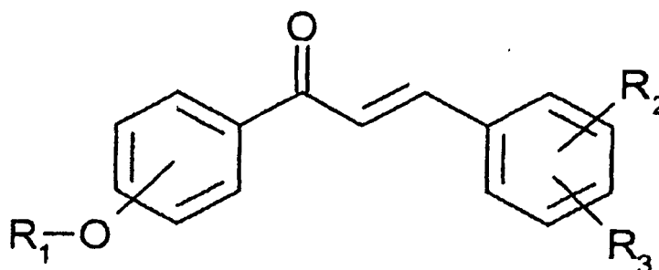
[Formule chimique 2]
