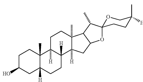
Sarsasapogenin
