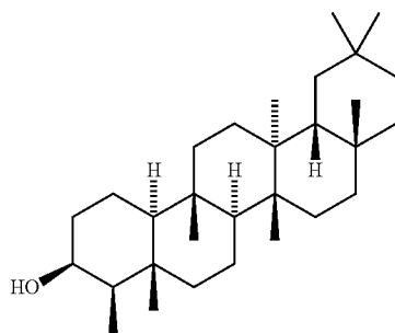
Epifriedelanol
