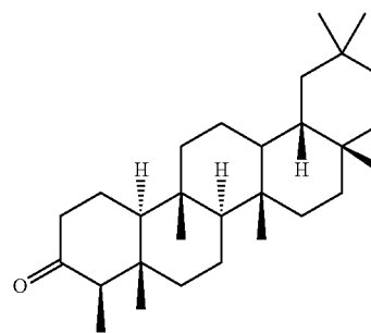
Friedelin
