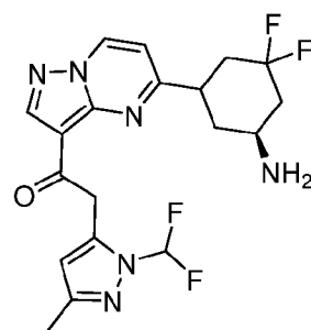
Merck 7
