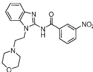
I-5409 (Sigma)
