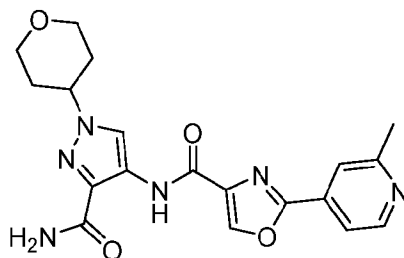
AS2444697
