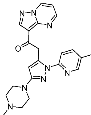
Merck 6
