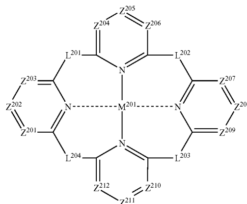
Formula (d)
