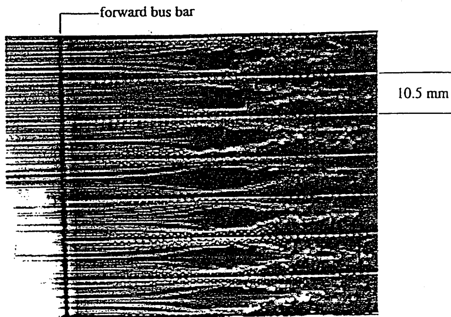
(a) E=3 kV rms, F=3 kHz
