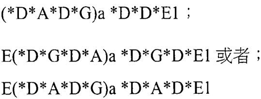
式 IV-VI
