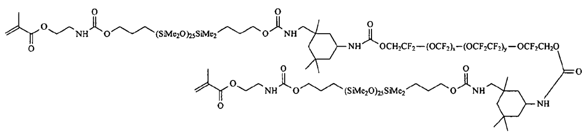
分子式 X
