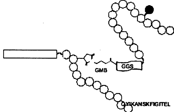
(301-311)-GMB-GGS-(E-421-436)
