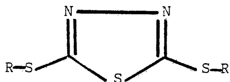
2,5-bis(hydrocarbylthio)-1,3,4-thiadiazole
