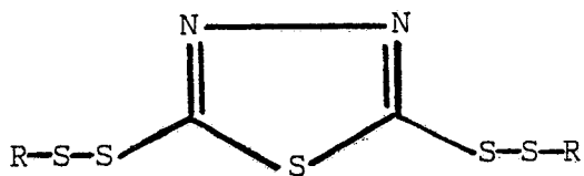
2,5-bis(hydrocarbyldithio)-1,3,4-thiadiazole
