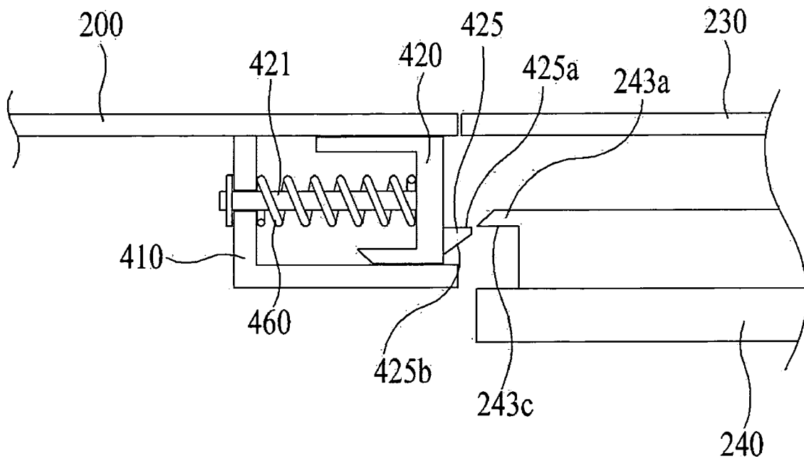
Fig. 17C
