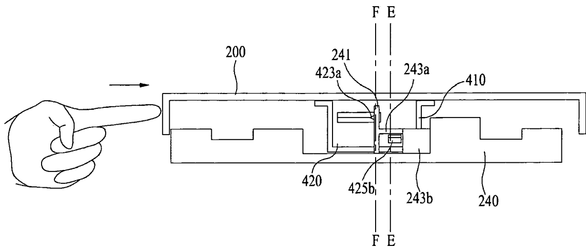
Fig. 17A
