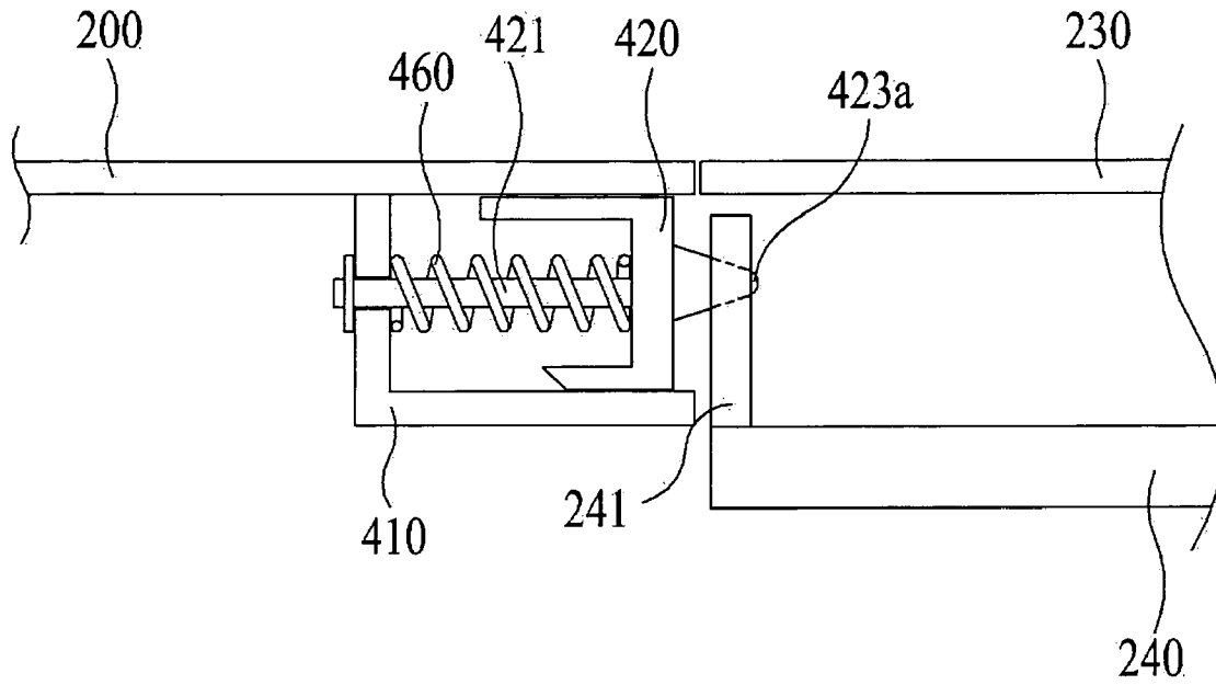
Fig. 17B
