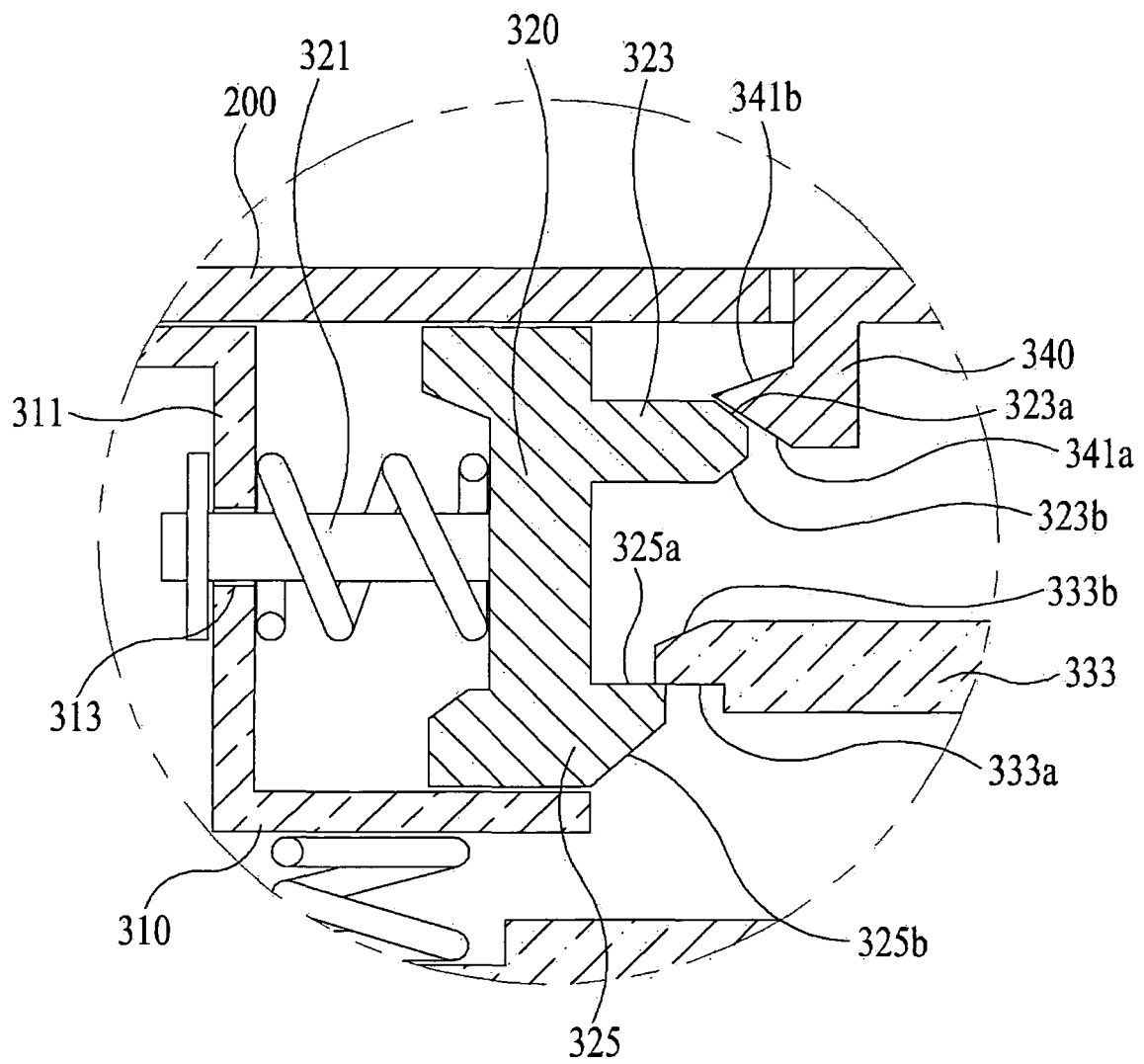
Fig. 9B
