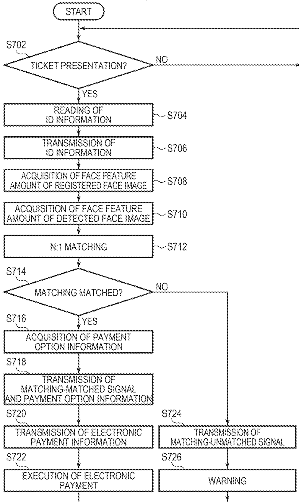
FIG. 24
