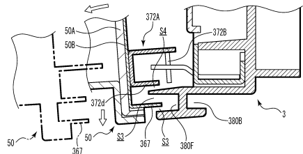
(A 3) 第1 開状態 (開放角度 : 約 5 度)
