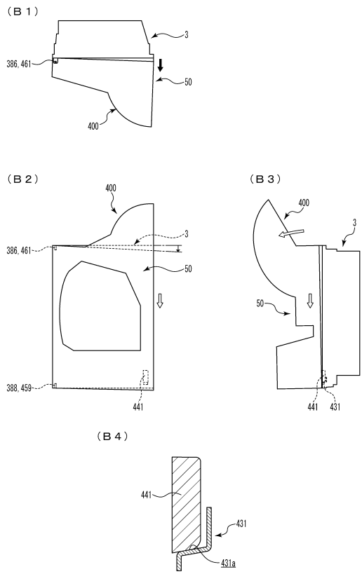
【図13-42】 開閉扉枠 [第1開状態 (開放角度: 約2度)]
