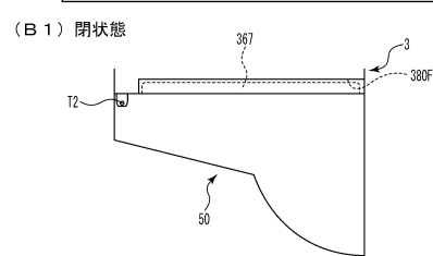
【図13-52】 開閉扉枠底部部品 (特定内部進入部品と被進入部品 / ドア枠所定部品と内枠所定部品)
