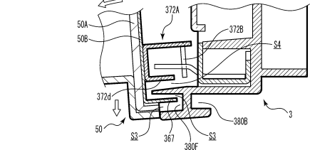
(A 2) 第1 開状態 (開放角度 : 約 2 度)
