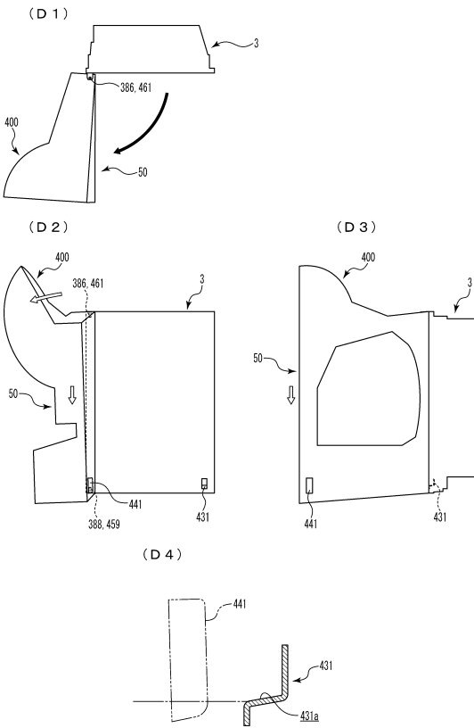
【図13-44】 開閉扉枠 [第2開状態 (開放角度: 約90度)]
