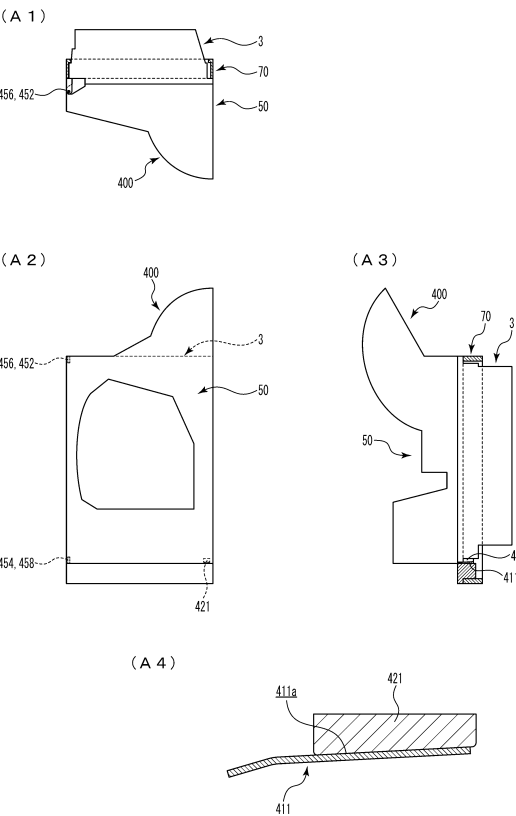
【図13-45】 遊技機用枠+開閉扉枠 [閉状態]
