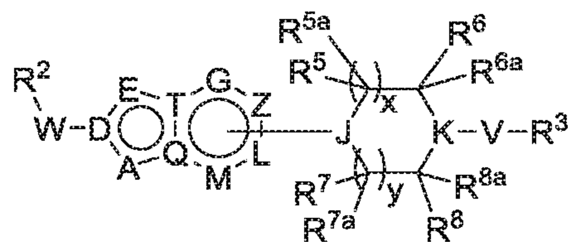
(VIIc)
