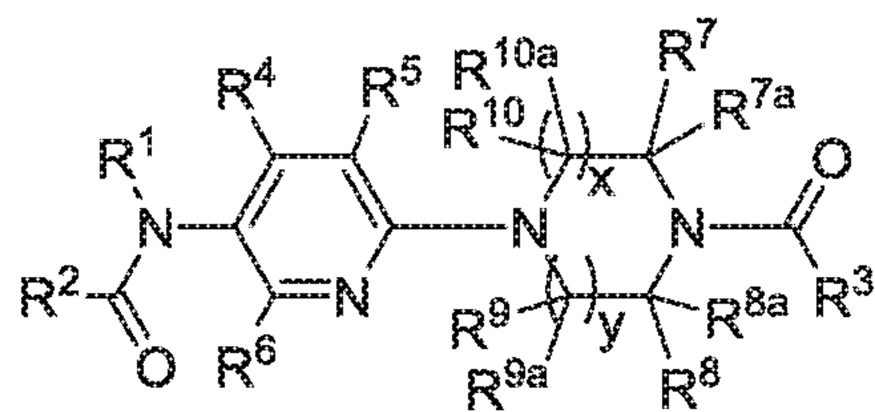
(IVcb)
