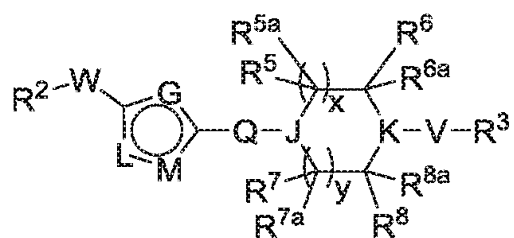
(Ia)
