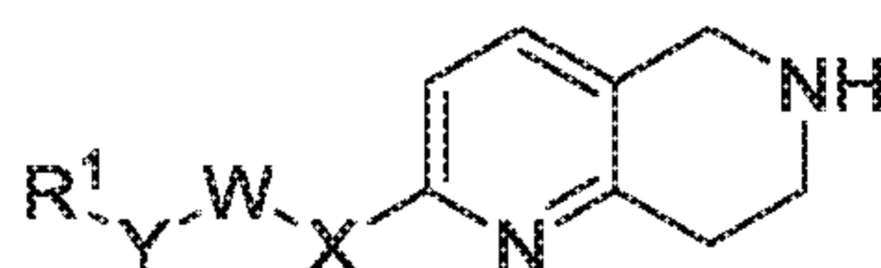
Formula LII
