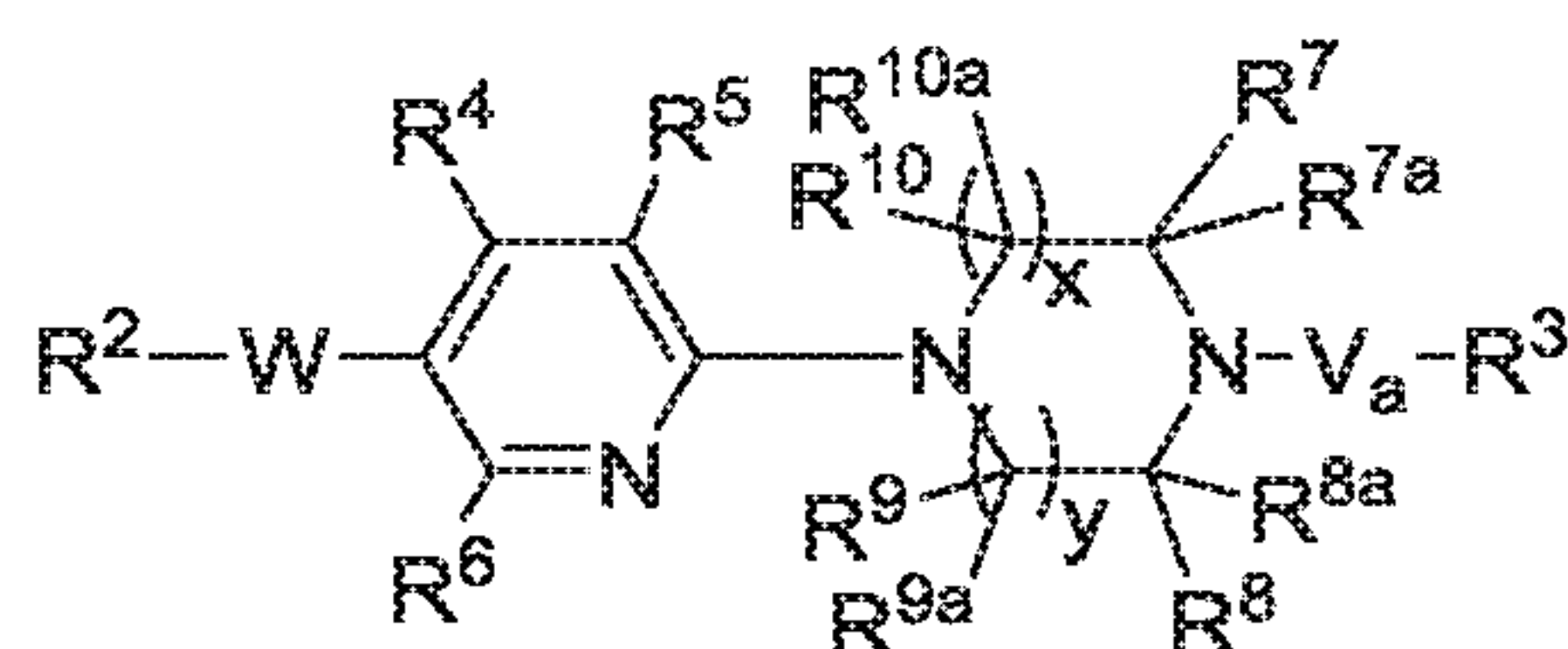
(IVaa)
