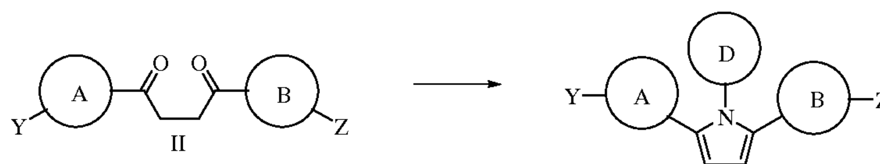
Scheme VI
