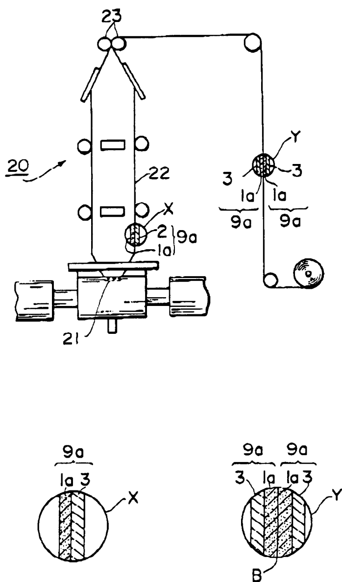
FIG. 29
