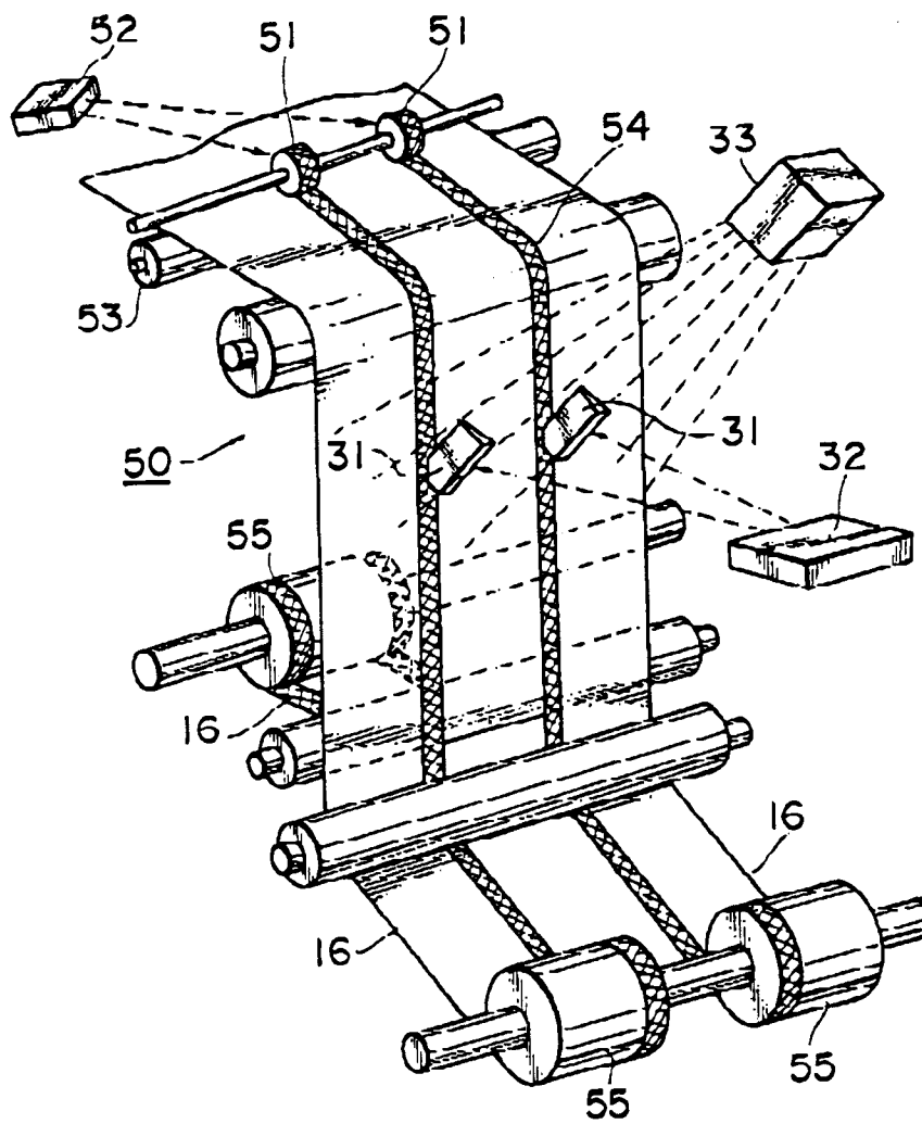
FIG. 34
