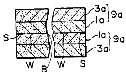
FIG. 25
