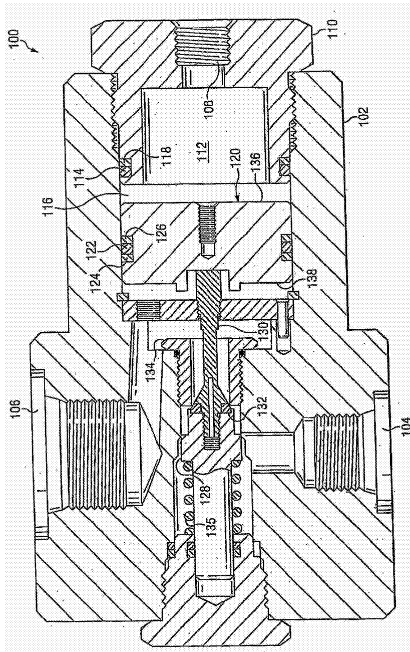
图1(现有技术)
