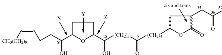
Mosinone A:
