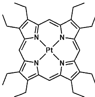
PtOEP
