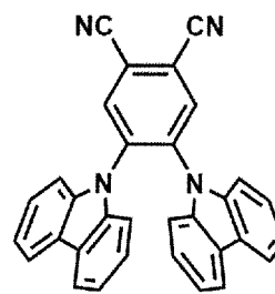
2CzPN
