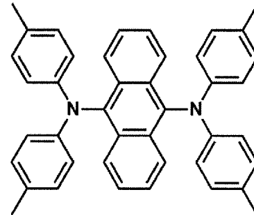
TTPA
