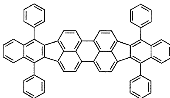
DBP
