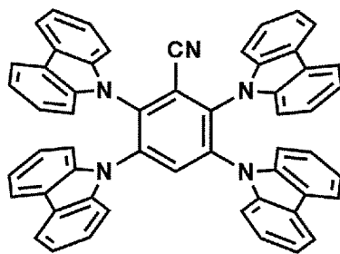
4CzBN
