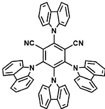
4CzIPN
