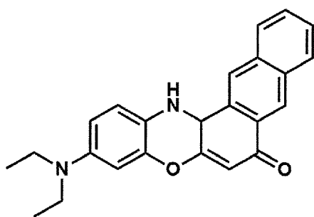
NileRed
