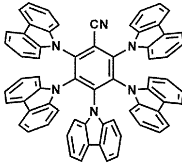
5CzBN
