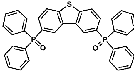
PPT
