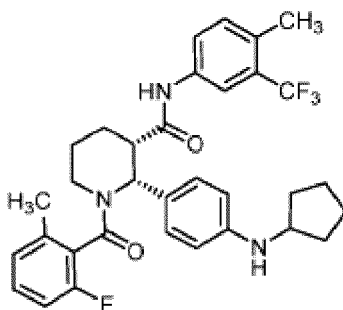
(Verbindung 1)
