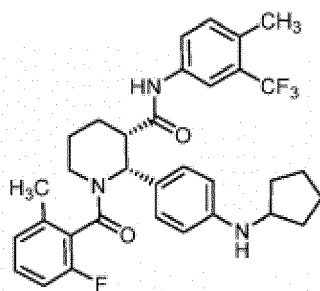
(Composé 1)
