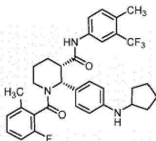
(Composé 1)
