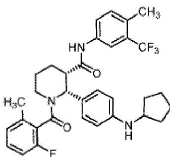
(Verbindung 1)
