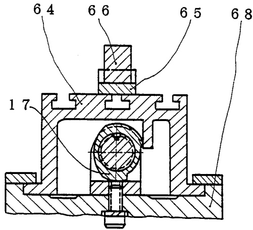
FIG. 9-II G-G
