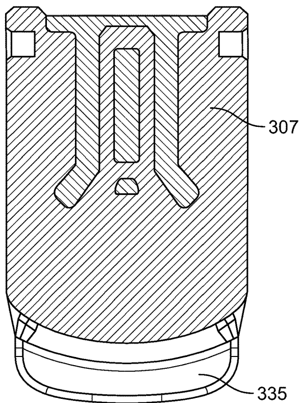
SECTION H-H FIG. 14E
