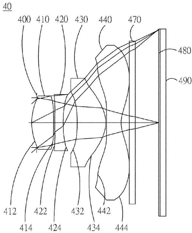
FIG. 4A
