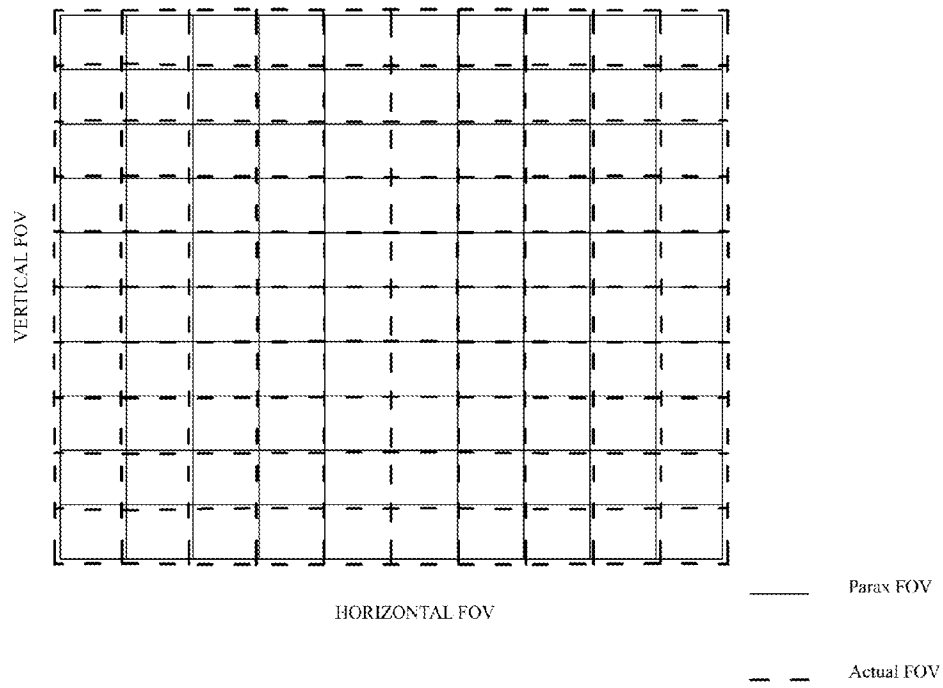
FIG. 5C
