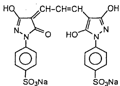
D-6
