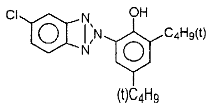
UV-4
