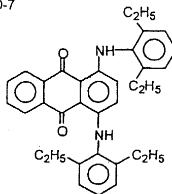
D-7
