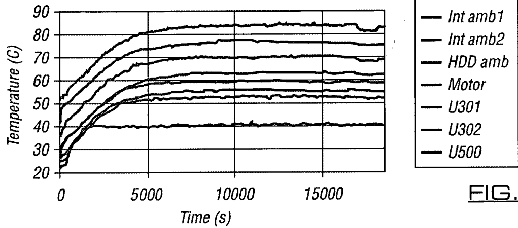
Temp test Power diss = 17.5W (puma) PVR3_11
