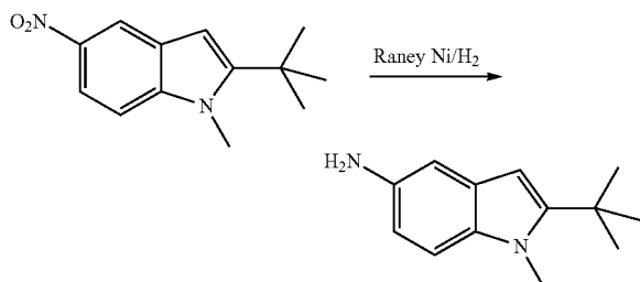
2-tert-Butyl-1-methyl-1H-indol-5-amine
