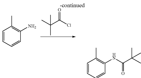
N-o-Tolylpivalamide
