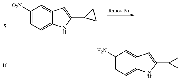
2-Cyclopropyl-1H-indol-5-amine
