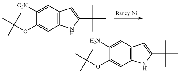
6-tert-Butoxy-2-tert-butyl-1H-indol-5-amine
