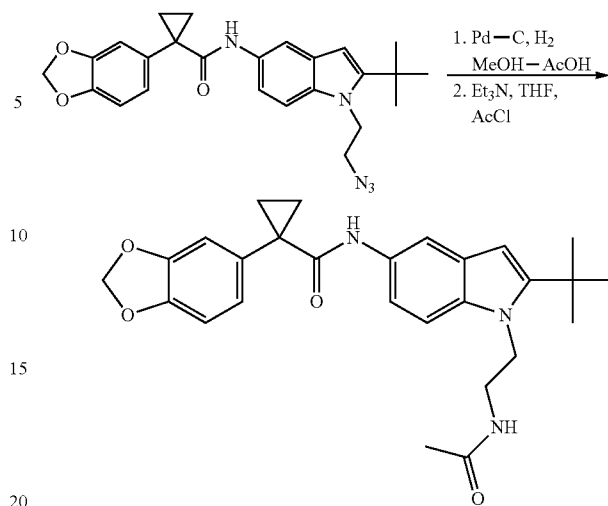
N-(1-(2-Acetamidoethyl)-2-tert-butyl-1H-indol-5-yl)-1-(benzo[d][1,3]dioxol-5-yl)cyclopropanecarboxamide
