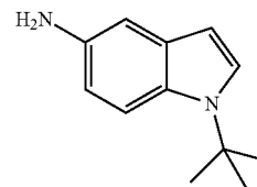
1-tert-Butyl-1H-indol-5-amine
