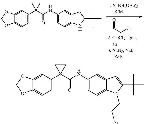
N-(1-(2-azidoethyl)-2-tert-butyl-1H-indol-5-yl)-1-(benzo[d][1,3]dioxol-5-yl)-cyclopropanecarboxamide
