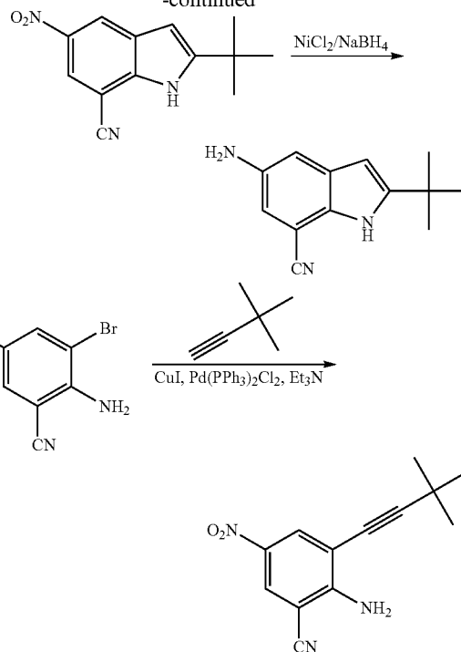
2-Amino-3-(3,3-dimethylbut-1-ynyl)-5-nitrobenzonitrile
