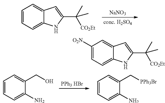
Triphenyl(2-aminobenzyl)phosphonium bromide
