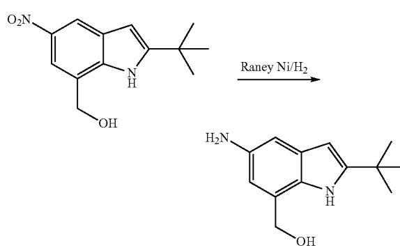
(5-Amino-2-tert-butyl-1H-indol-7-yl)methanol
