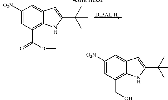
(2-tert-Butyl-5-nitro-1H-indol-7-yl)methanol
