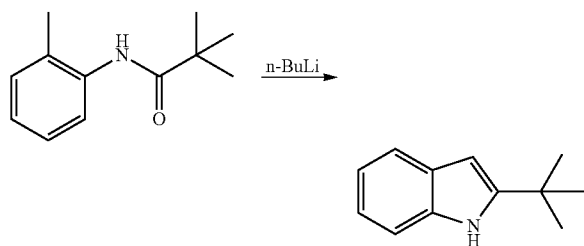
2-tert-Butyl-1H-indole
