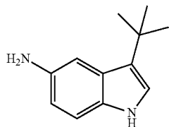
3-tert-Butyl-1H-indol-5-amine
