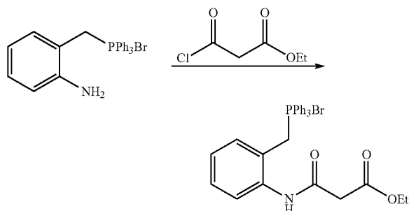
Triphenyl((ethyl(2-carbamoyl)acetate)-2-benzyl)phosphonium bromide
