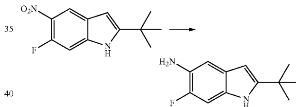
2-tert-Butyl-6-fluoro-1H-indol-5-amine
