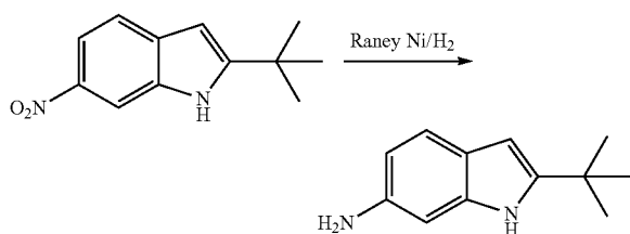
2-tert-Butyl-1H-indol-6-amine
