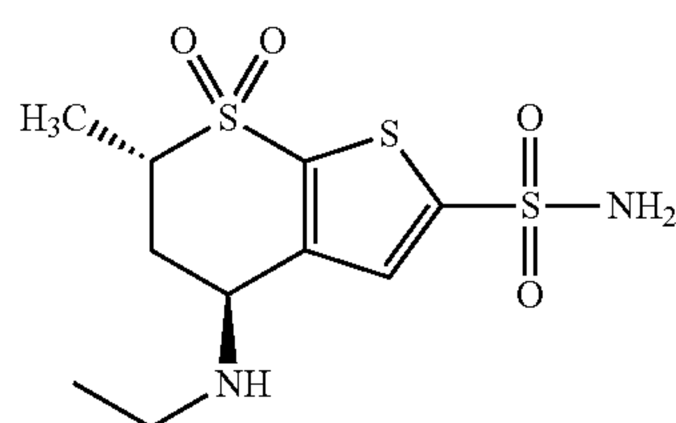
Dorzolamide
