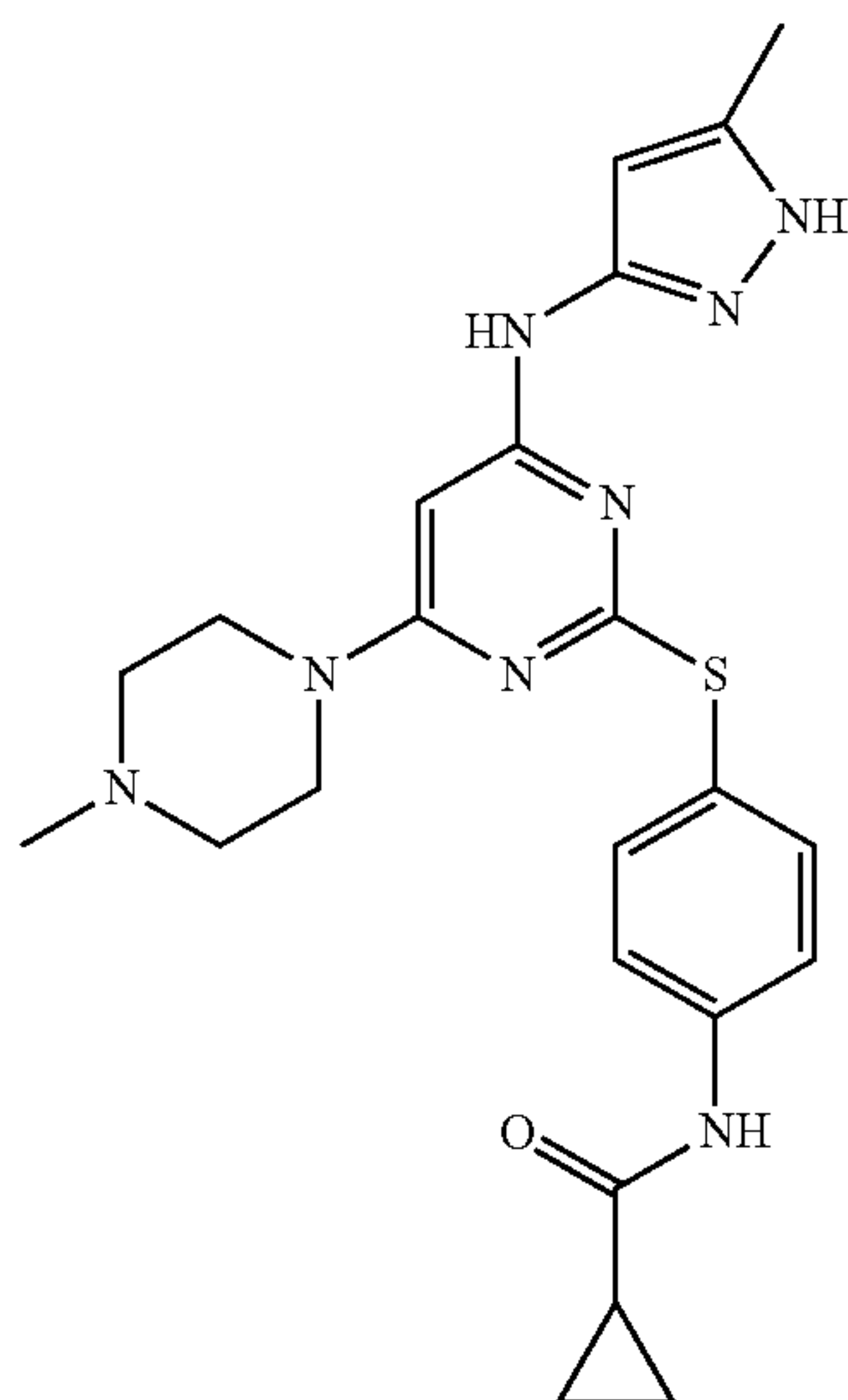
Tozasertib
