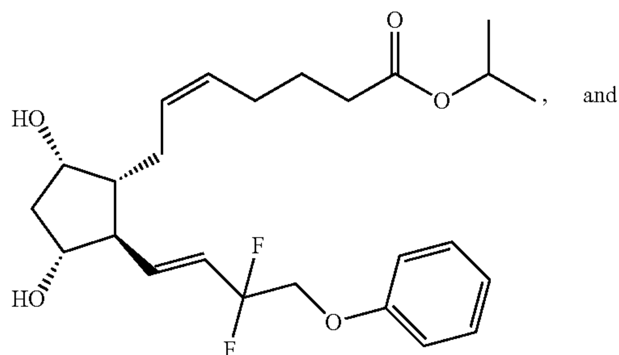
Tafluprost
