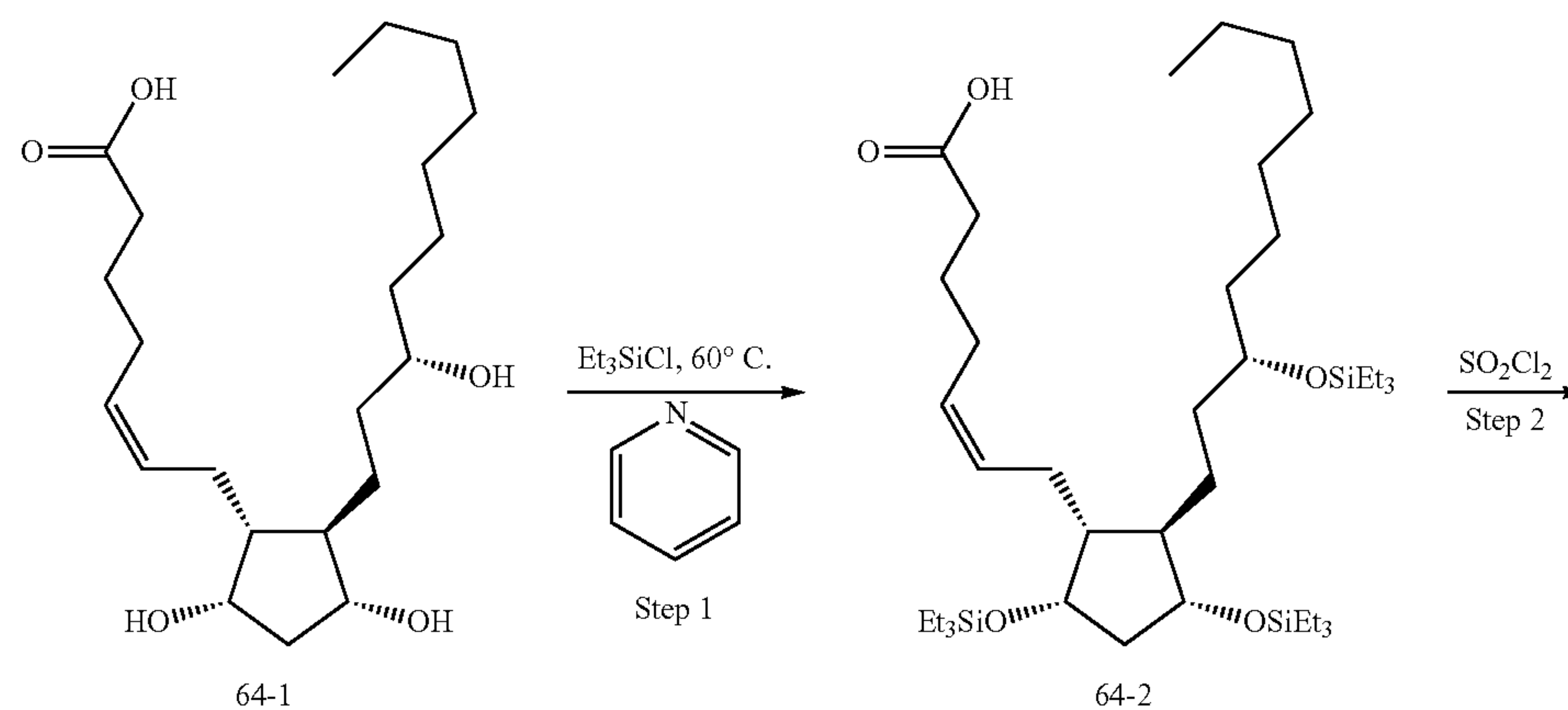
Scheme 64:
