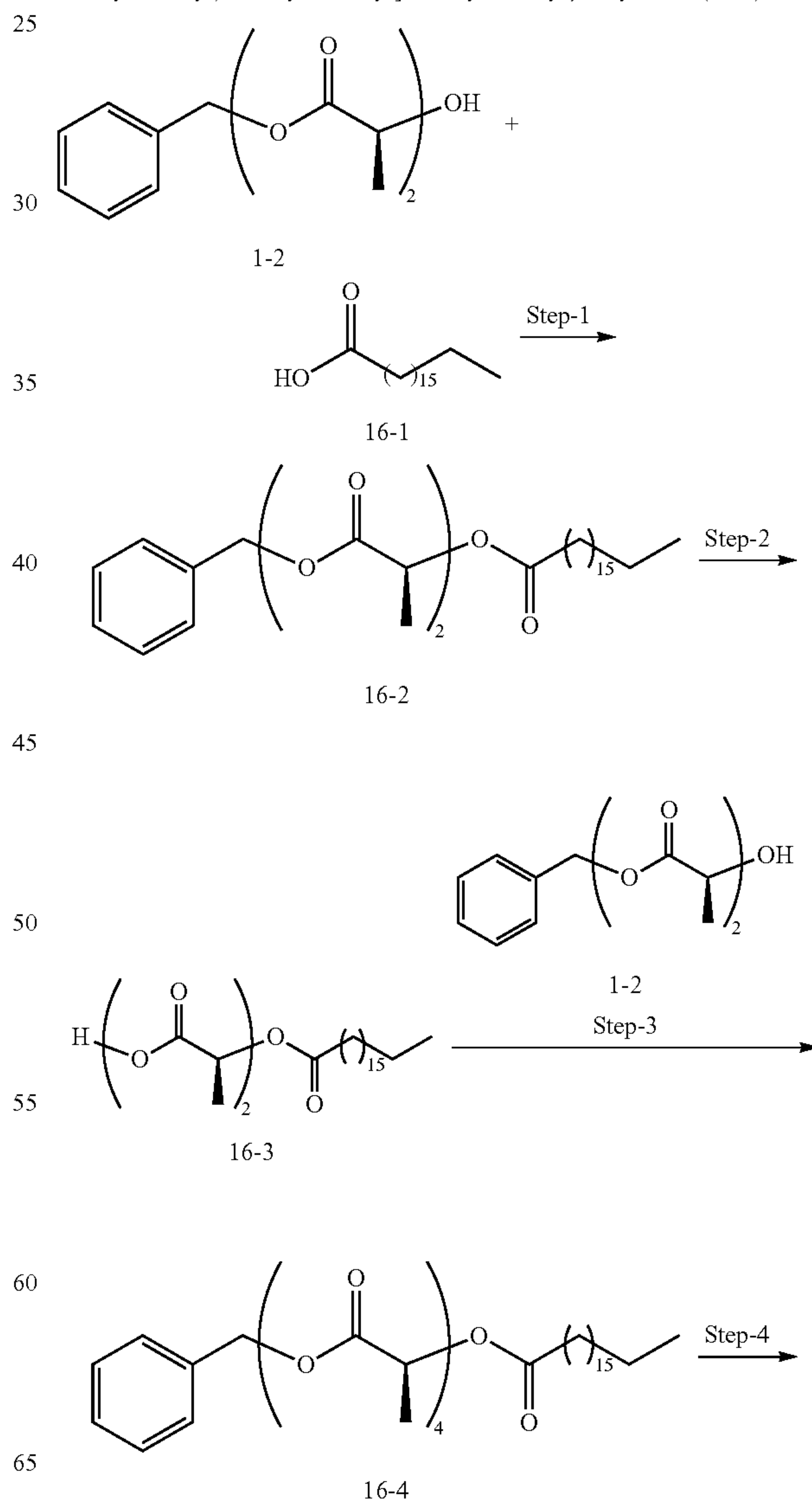
Scheme 16: Octadecanoic acid (S)-1-((S)-1-((S)-1-((S)-1-carboxy-ethoxycarbonyl)-ethoxy carbonyl]-ethoxycarbonyl)-ethyl ester (16-5):
