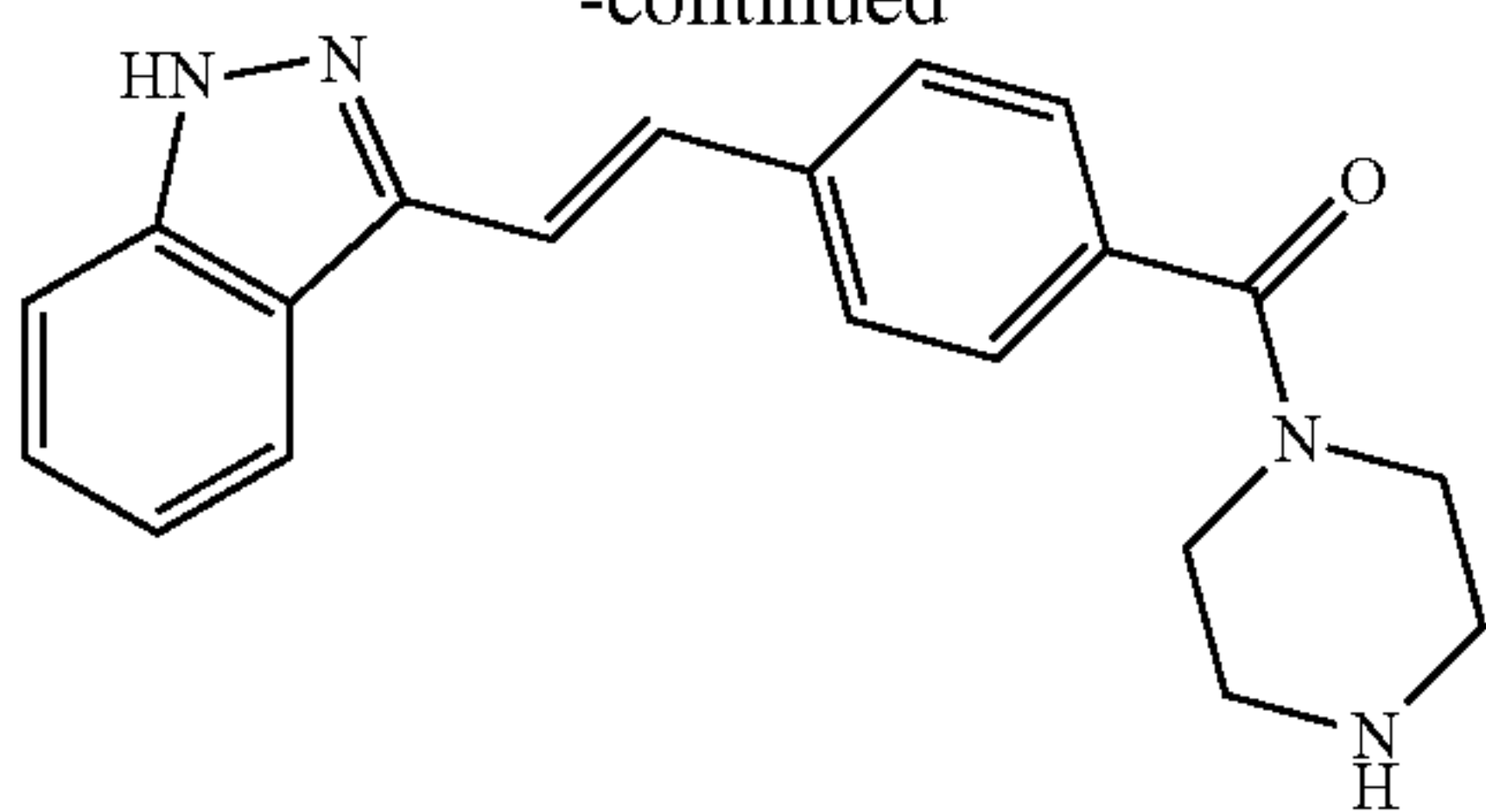
KW-2449
