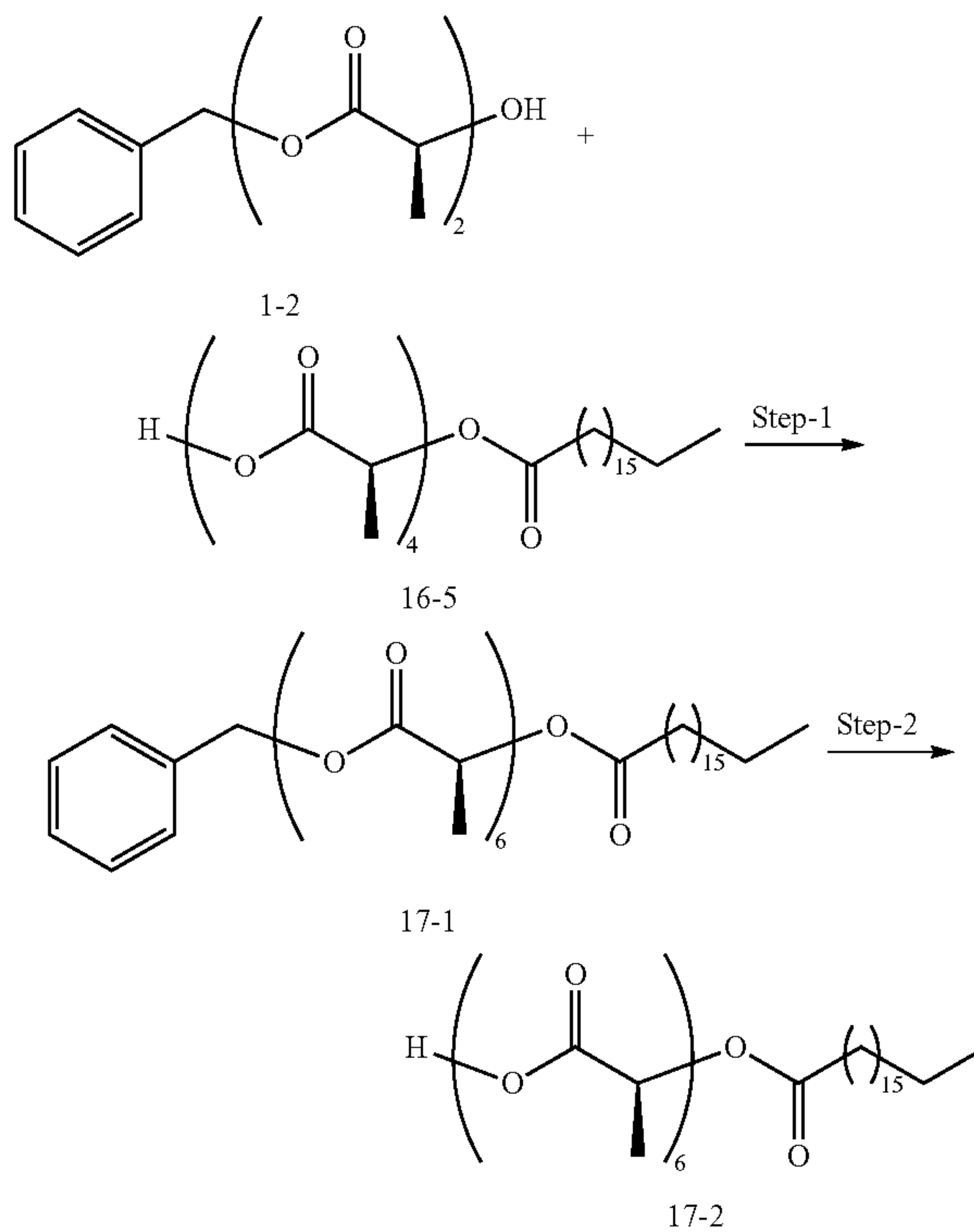
Scheme 17: Octadecanoic acid (S)-1-[(S)-1-((S)-1-((S)-1-[(S)-1-((S)-1-carboxy-ethoxycarbonyl)-ethoxycarbonyl]-ethoxycarbonyl)-ethoxycarbonyl)-ethoxycarbonyl]-ethyl ester(17-2):
