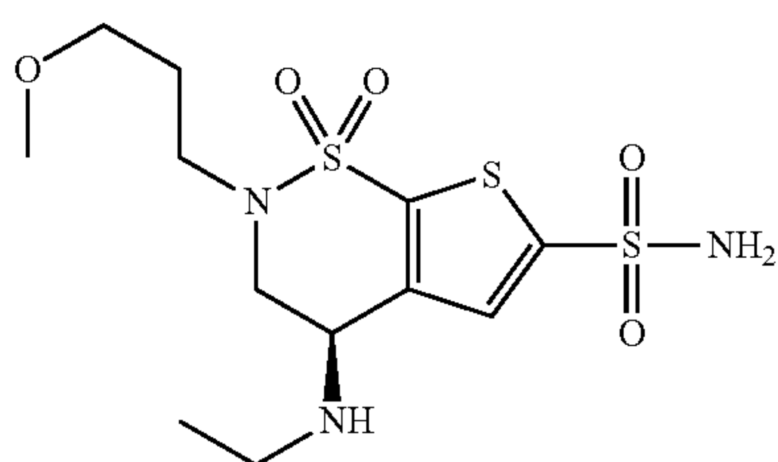
Brinzolamide
