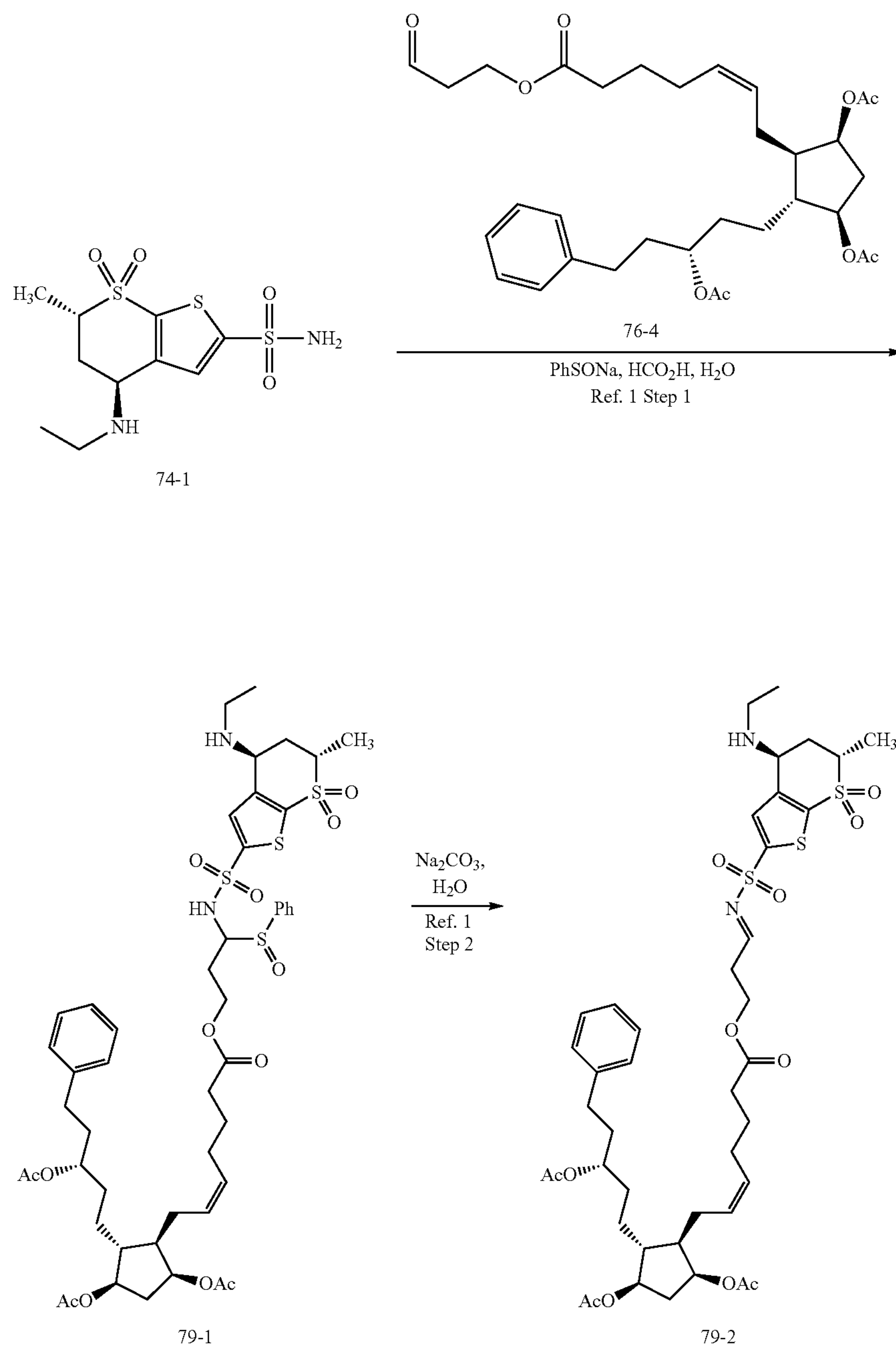
Scheme 79:
