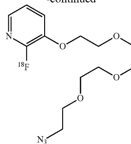
Synthesis of [ 18 F]-3-(2-(2-(2-azidoethoxy)ethoxy)ethoxy)-2-fluoropyridine
