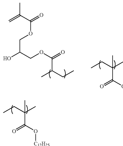
Macromonomer M-5
