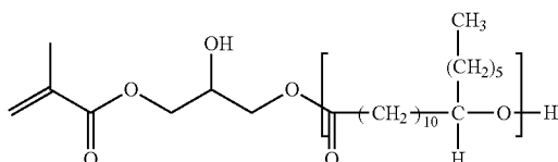
Macromonomer M-2
