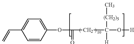
Macromonomer M-3
