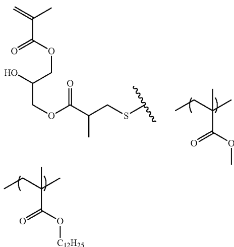
Macromonomer M-1
