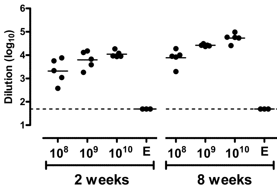
B) Ad35-RSV.F
