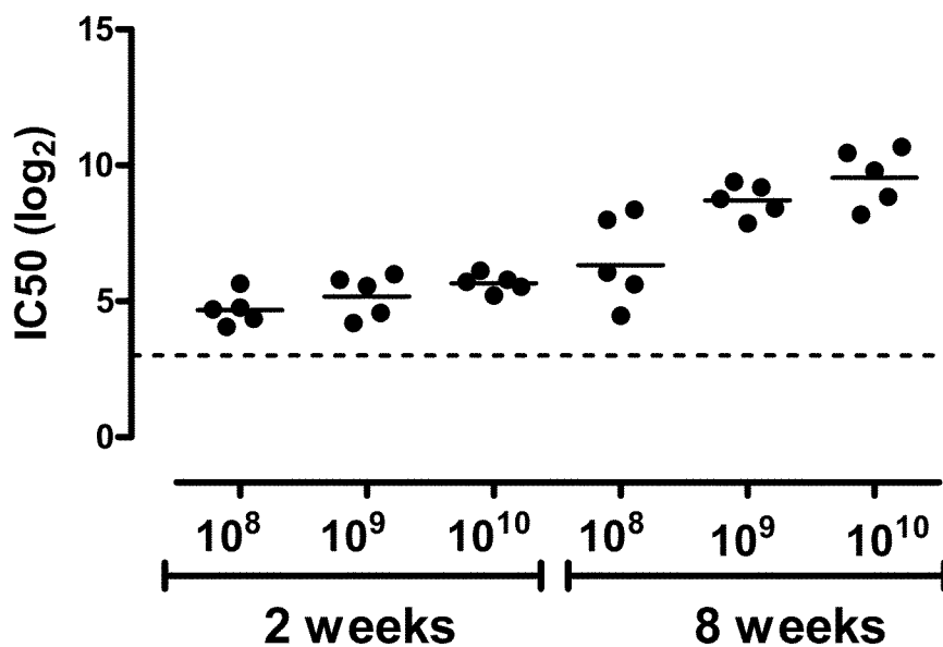
A) Ad26-RSV.F
