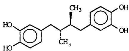
Nordihydroguaiaretic Acid
