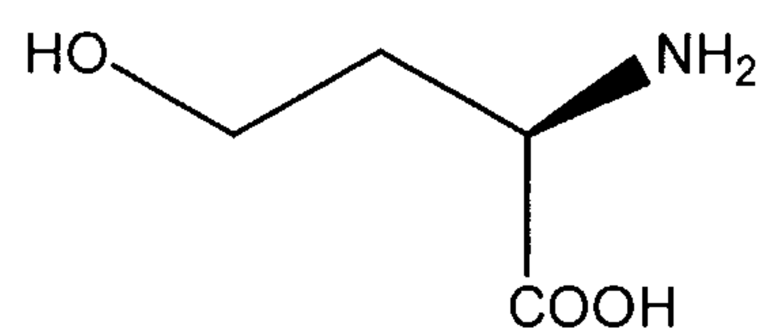
D-homoserine
