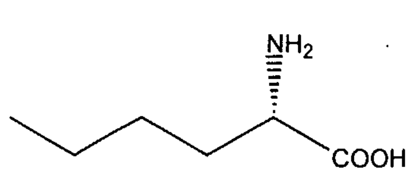
L-norleucine
