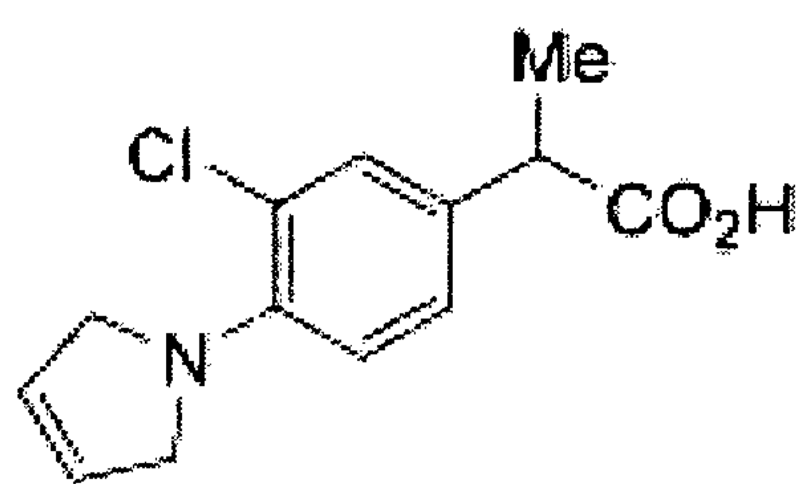
Pirprofen
