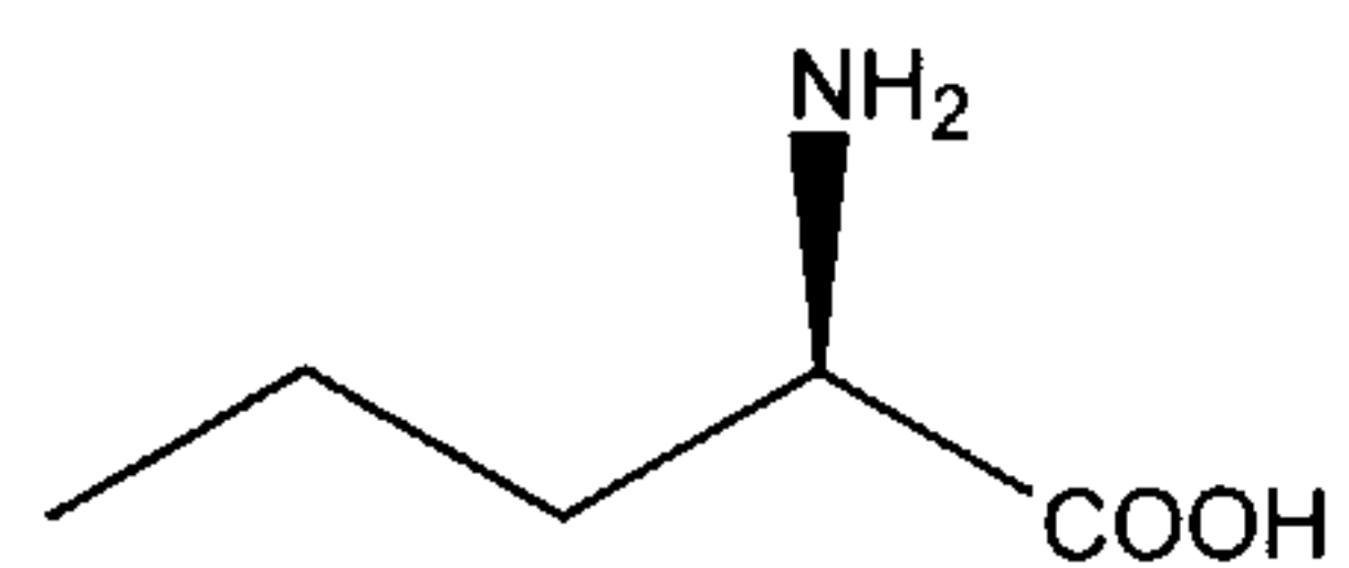
D-norvaline
