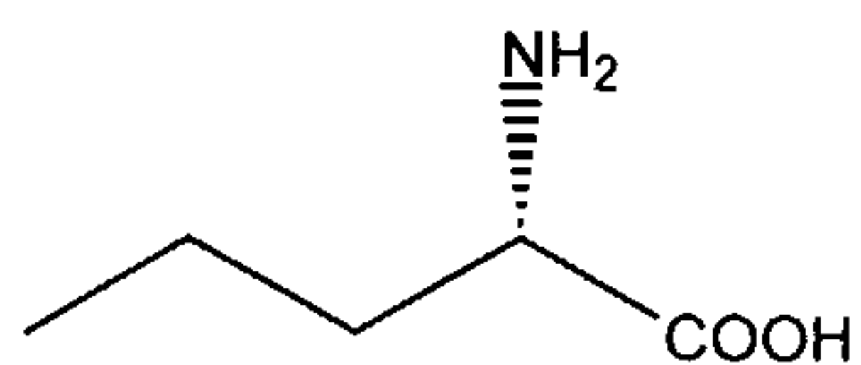
L-norvaline
