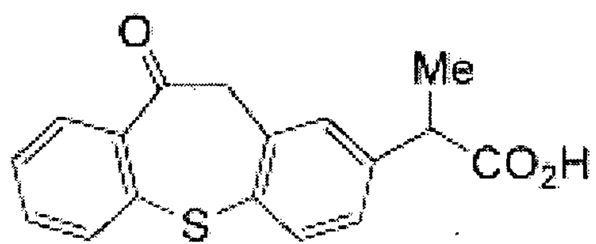
Zaltoprofen
