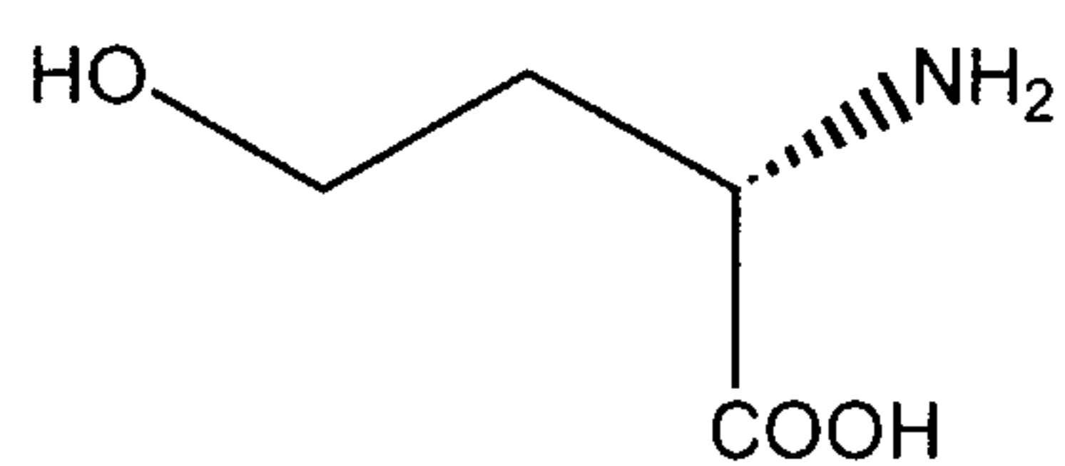
L-homoserine
