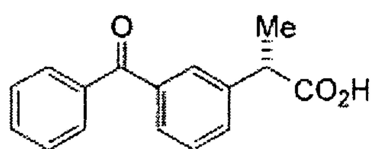
Dexketoprofen
