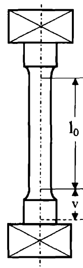
Fig. 6. Alungirea epruvetei
