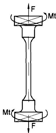
Fig. 2. Epruvetă sollicitată la tracțiune și torsiune
