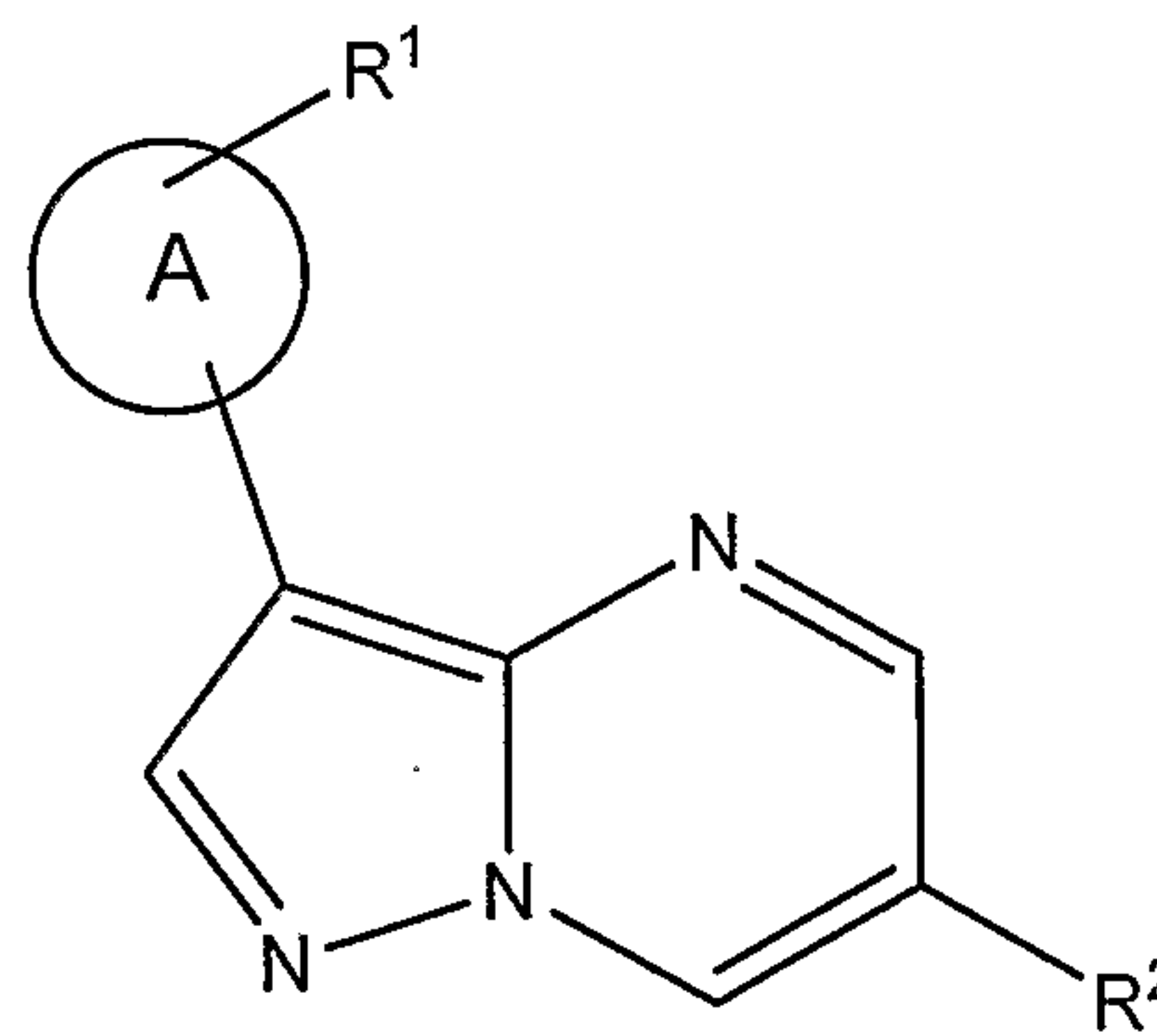
(Id)
