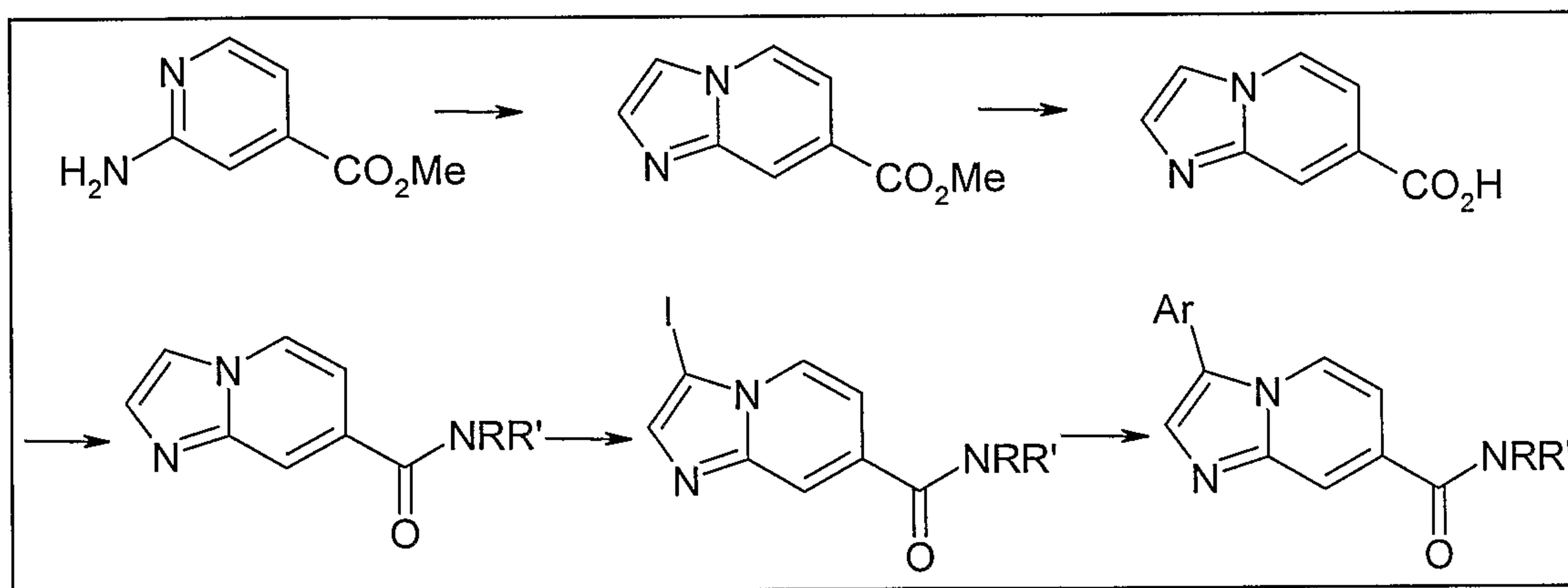
Scheme 1A
