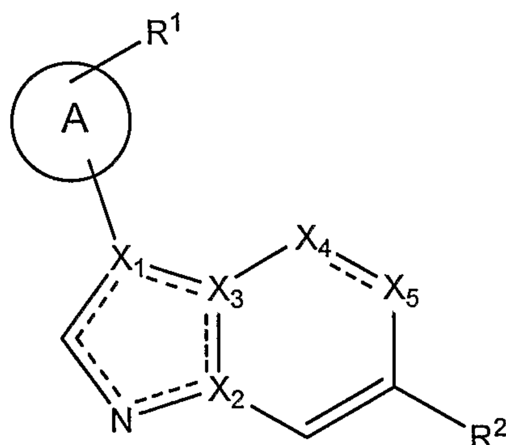
(Ia)
