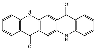
5,12-dihydroquinu[2,3-b]acridine-7,14-dione
