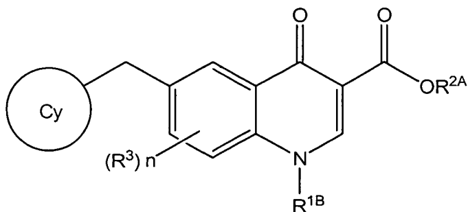
[I-4]
