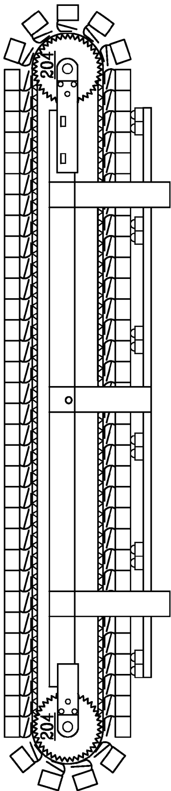
SECTION B-B FIG. 4
