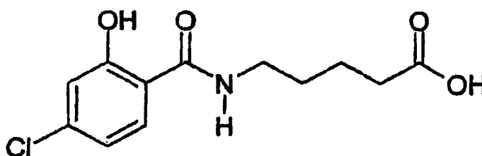
Verbindung 1
