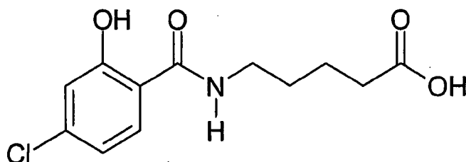
composé 1
