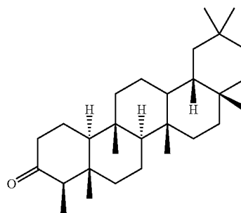
Friedelin
