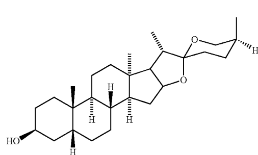
Sarsasapogenin
