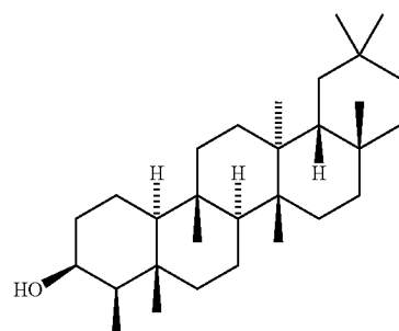
Epifriedelanol
