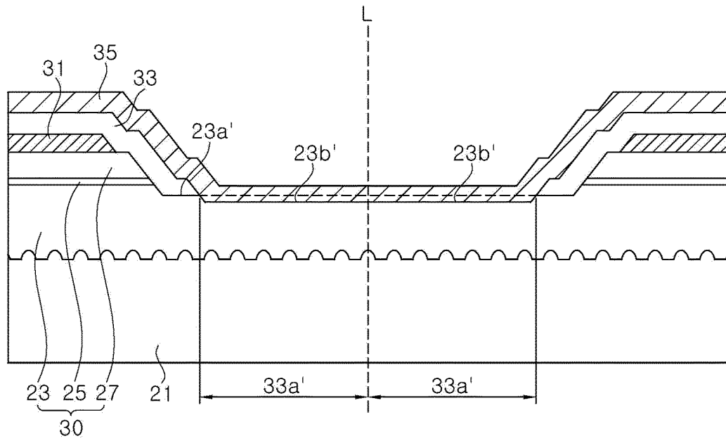
【FIG. 7D】
