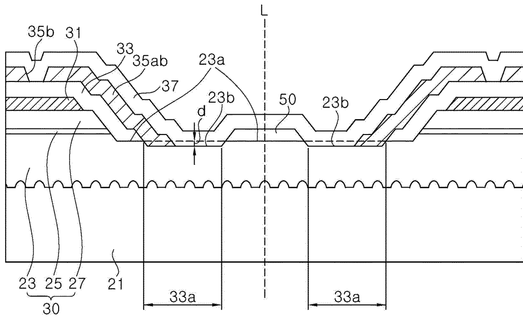
【FIG. 6E】
