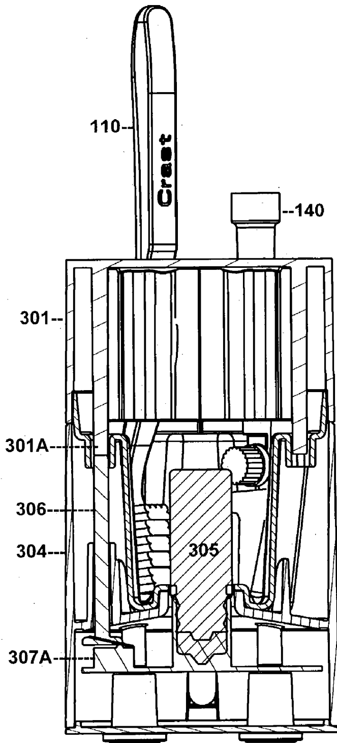
SECTION A-A
