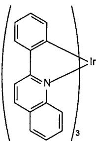
Ir(pq) 3
