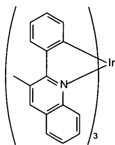
Ir(3-Mepq) 3
