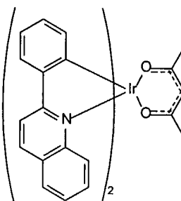
Ir(pq) 2 (acac)
