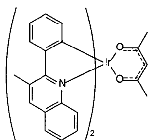
Ir(3-Mepq) 2 (acac)
