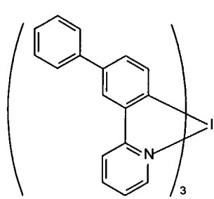
Ir(Phppy) 3
