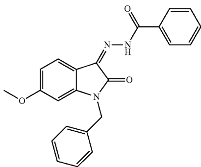
A) 1-benzyl-6-methoxy-isatin
