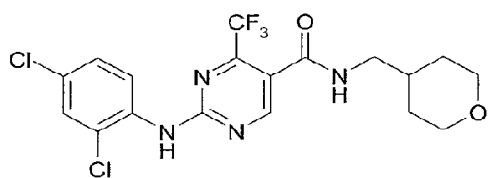
GW842166X
