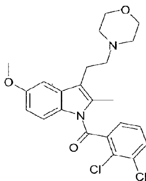
GW405833 (L768242)
